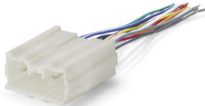
CÓDIGO: 40123 CHICOTE DE LIGAÇÃO P/ PAJERO TODOS OS MODELOS ATÉ 2008
